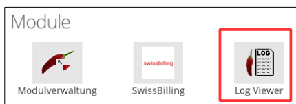
Abbildung 7: Log-Viewer Modul
