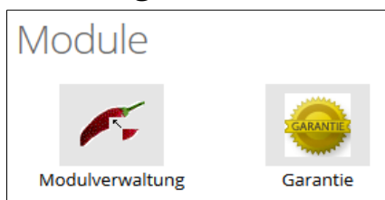
Abbildung 1: PepperShop Module
